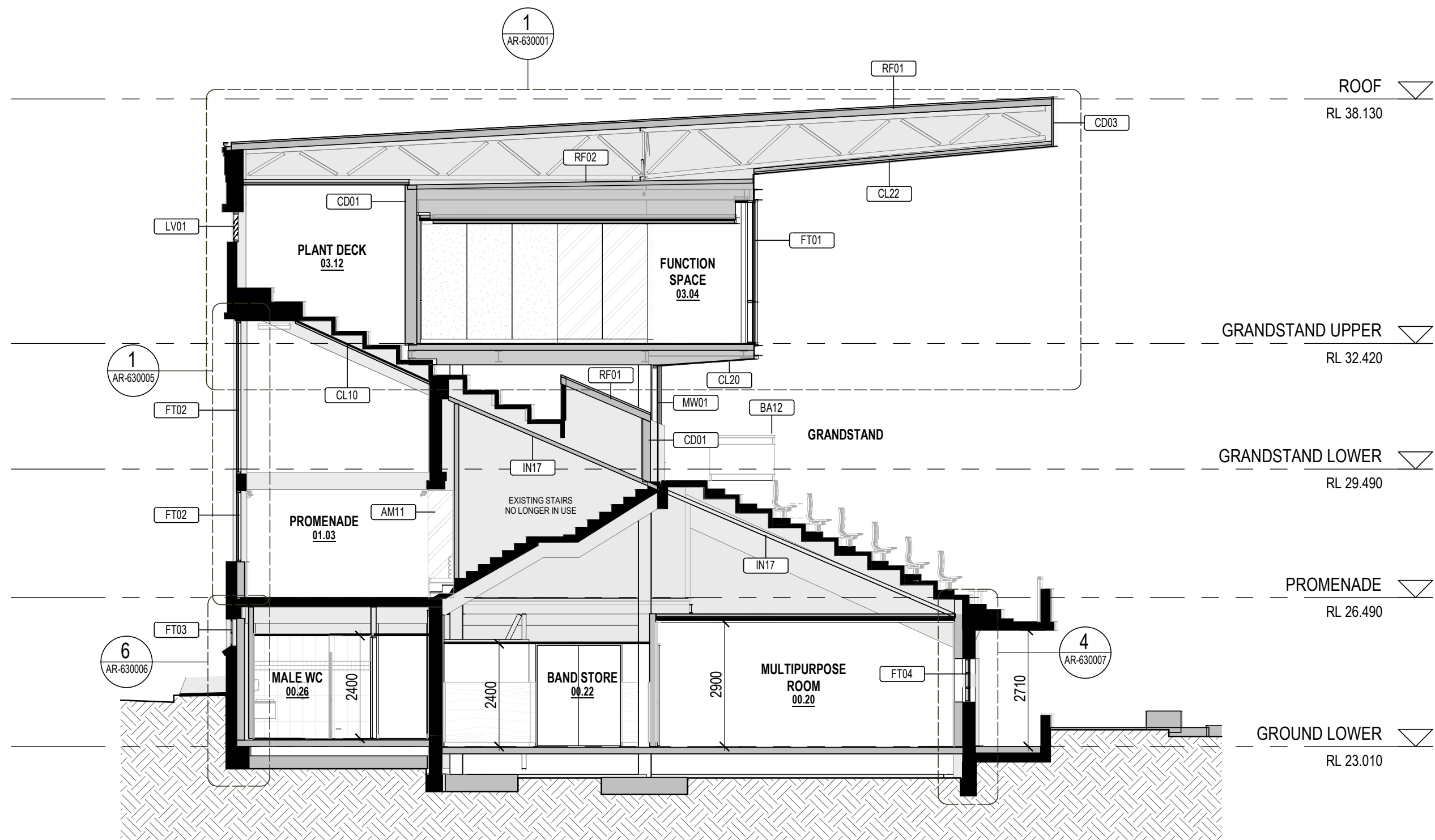
5 CROSS SECTION 5 SCALE: 1:100
