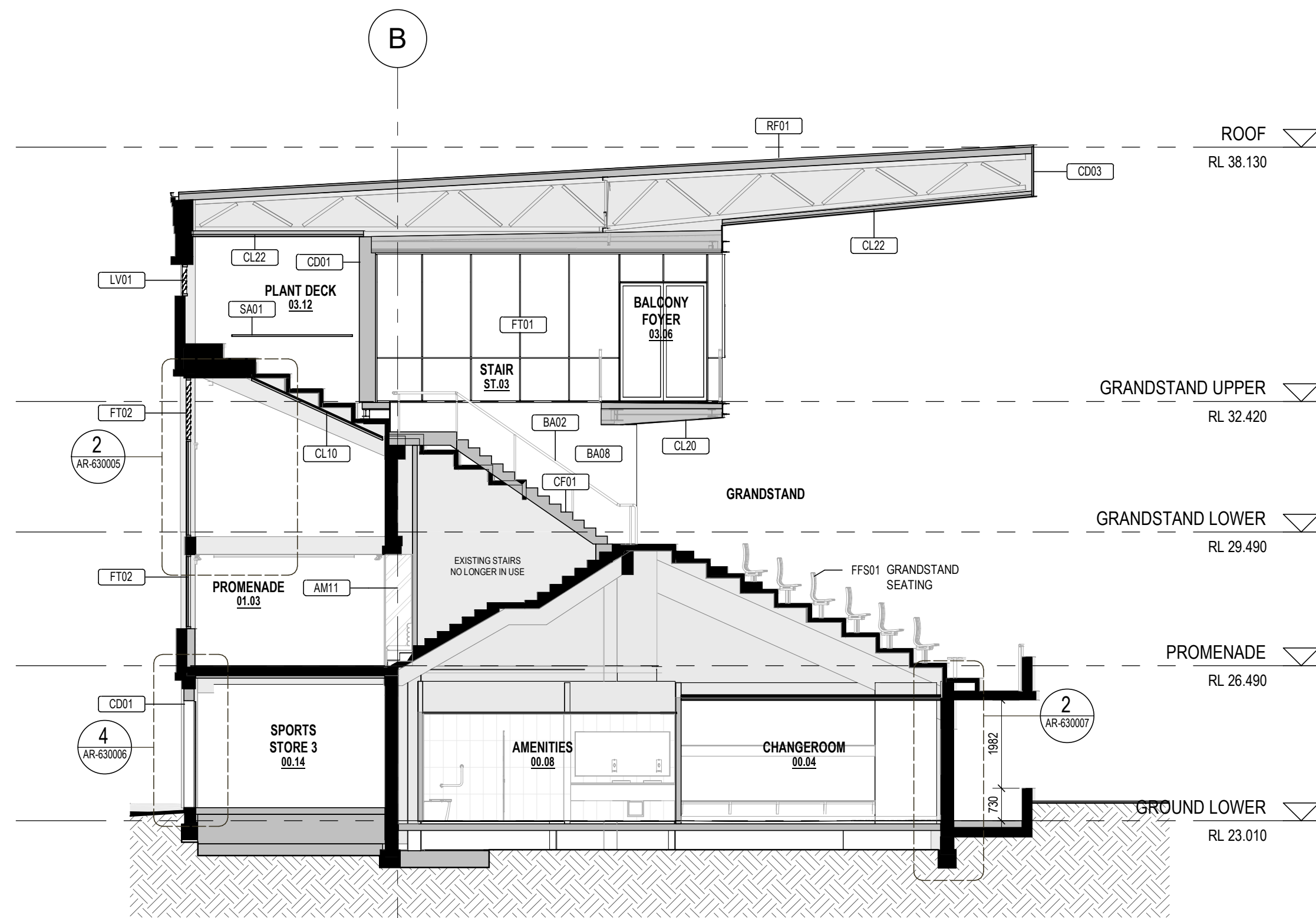
3 CROSS SECTION 3 SCALE: 1:100
