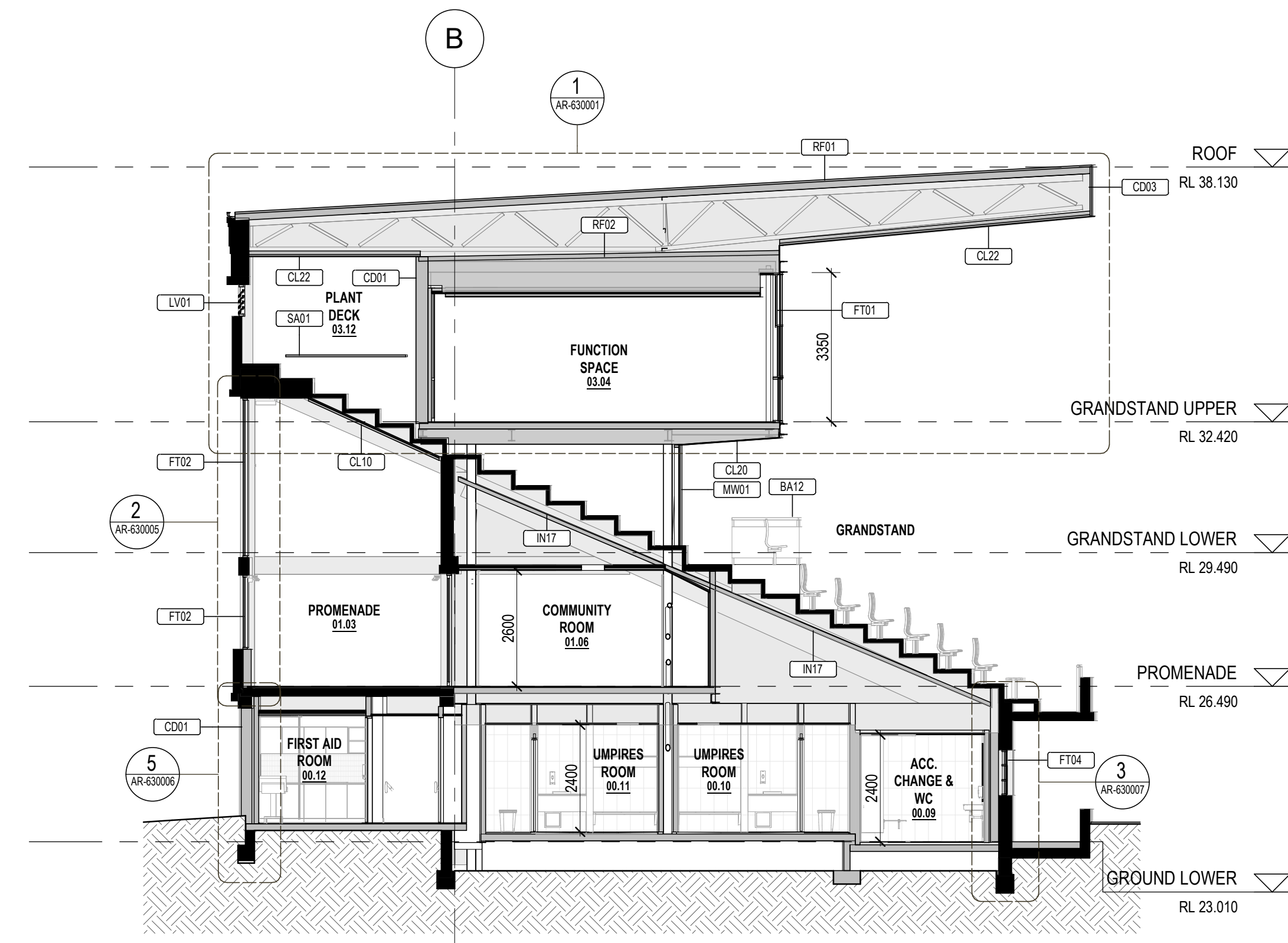
4 CROSS SECTION 4 SCALE: 1:100
