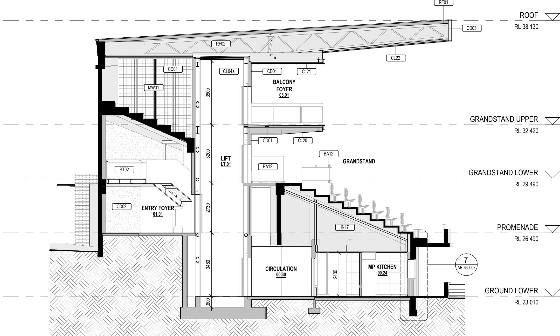
8 CROSS SECTION 8 SCALE: 1:100
