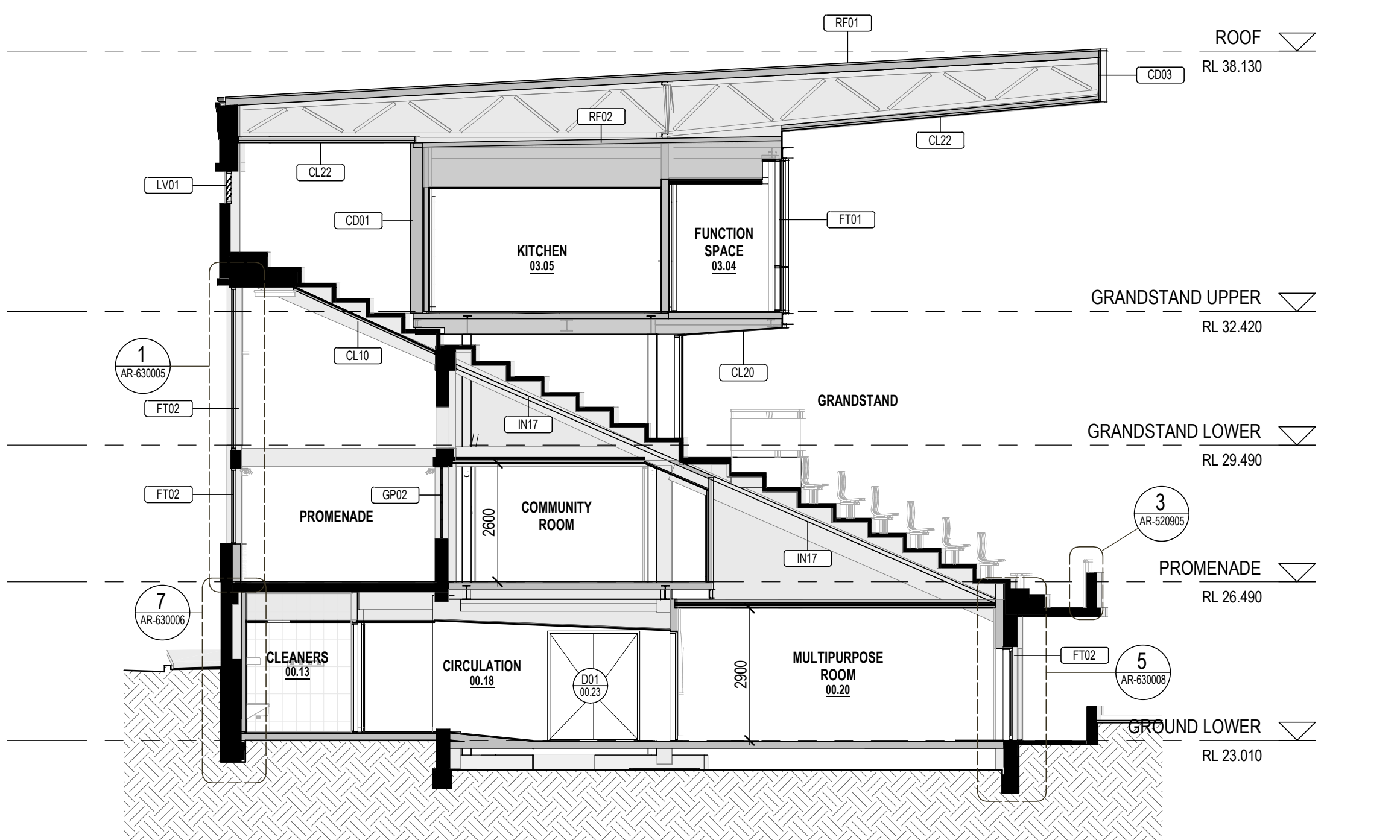
6 CROSS SECTION 6 SCALE: 1:100
