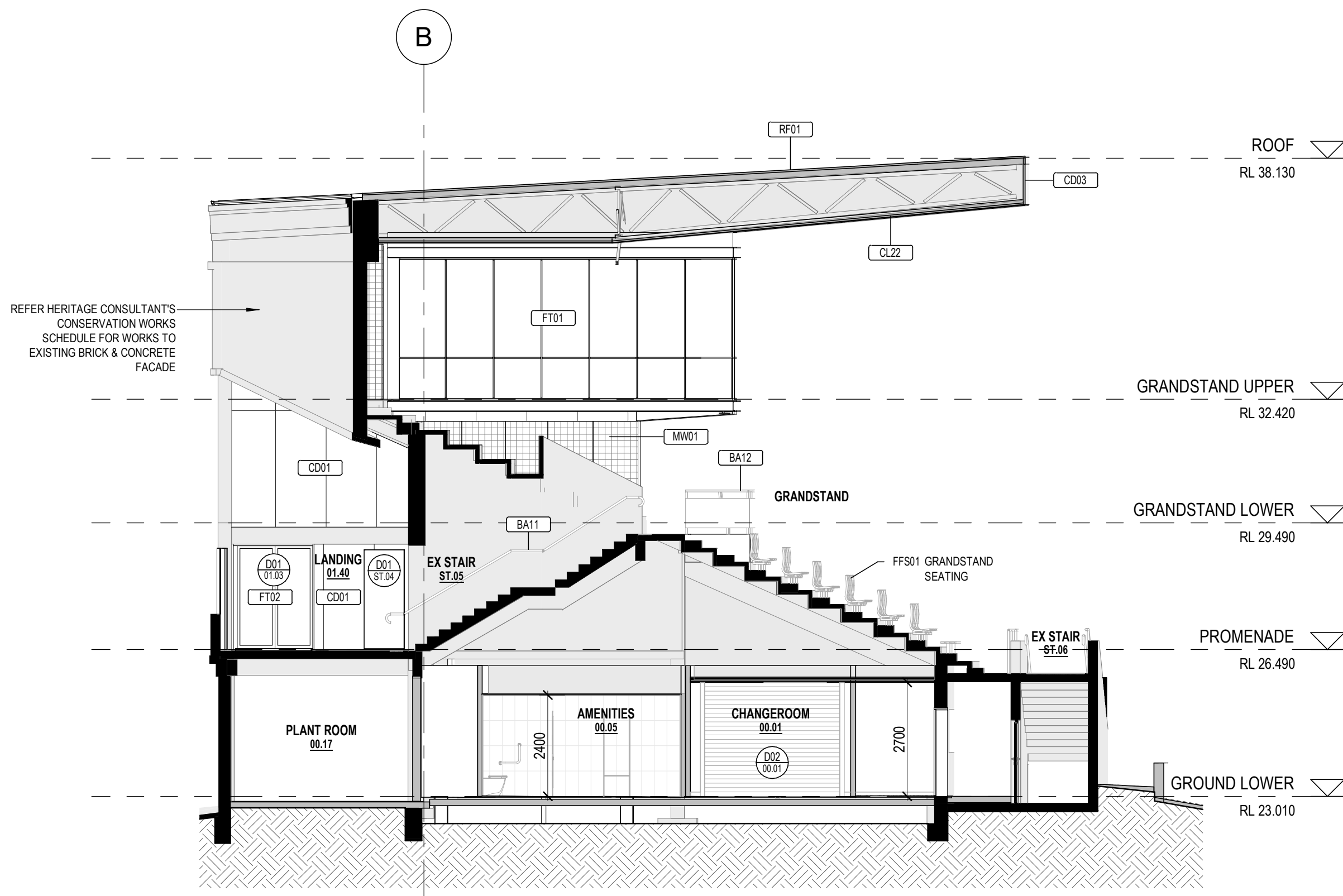
1 CROSS SECTION 1 SCALE: 1:100
