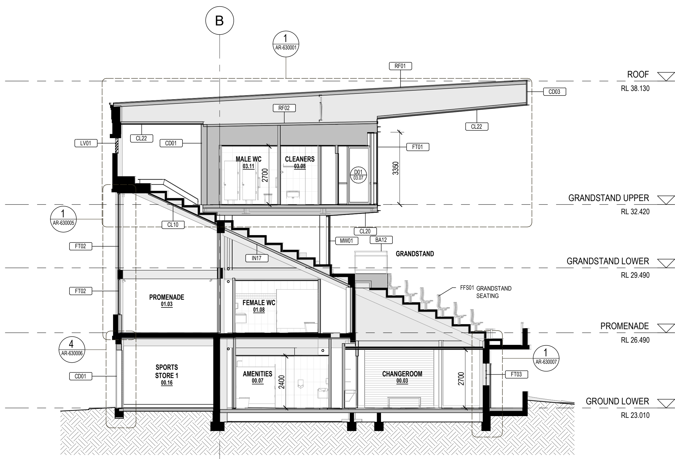
2 CROSS SECTION 2 SCALE: 1:100
