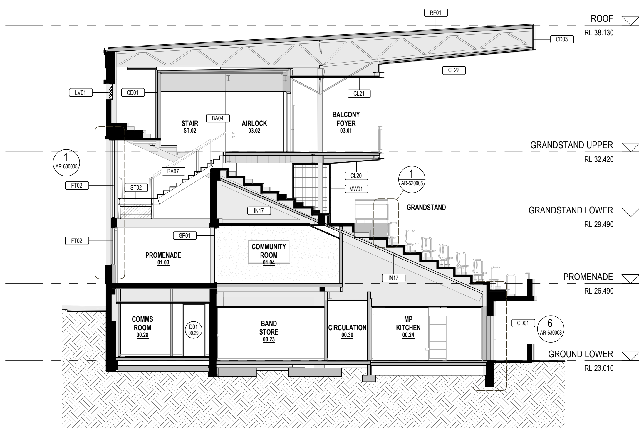
7 CROSS SECTION 7 SCALE: 1:100
