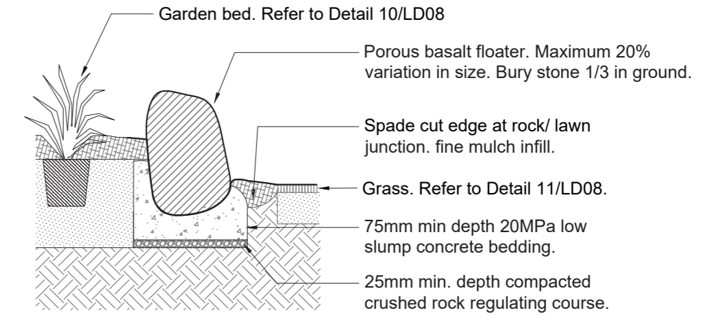
Garden Bed Edge Detail
