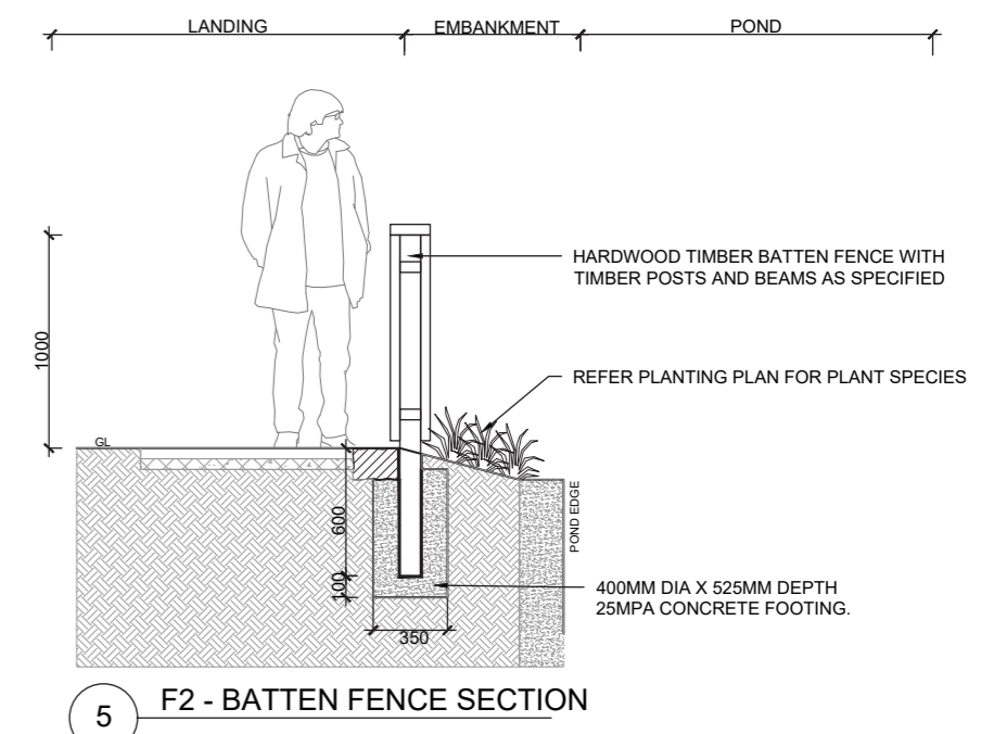
5 F2 - BATTEN FENCE SECTION
